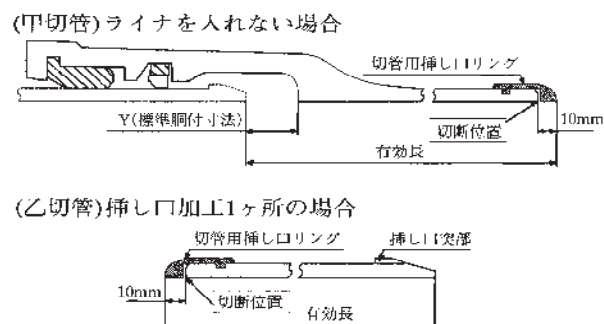
図 3.3.84 切断位置と有効長
