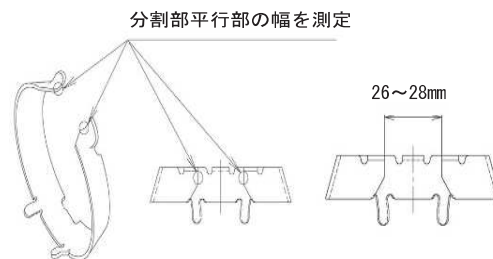
図 3.3.126 ロックリングの再装着時の確認
