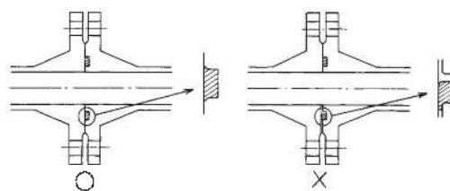
図 3.3.148 ガスケットの正しい位置
