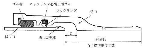
図 3.3.74 NS形継手の構造（直管）
