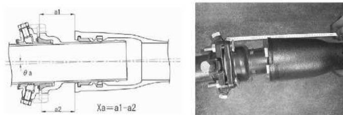
図 3.3.123 曲げ角度の確認方法
