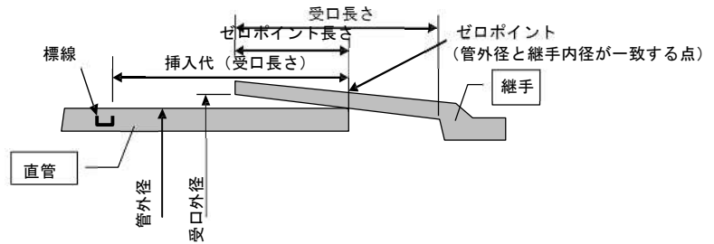
図 3.3.156 ゼロポイントの確認
