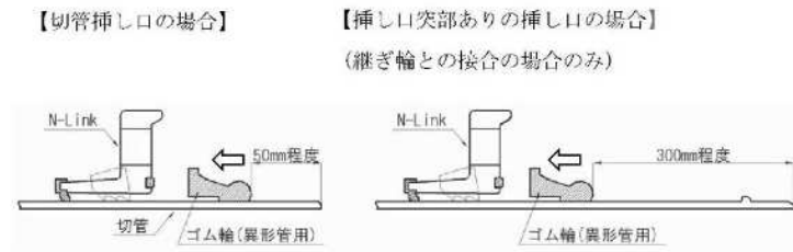
図 3.3.117 ゴム輪の預け入れ
