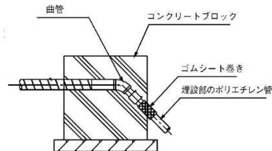
図 3.3.152 防護コンクリートによる対策
