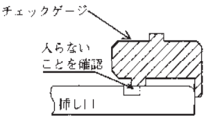
図 3.3.86 挿し口端面から溝までの距離の確認
