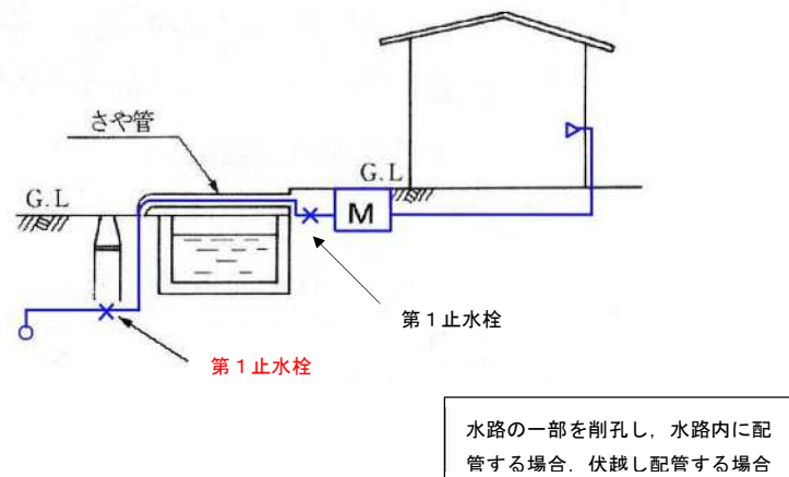
図 4.1.9 公道上等に設置する第1止水栓の設置例
