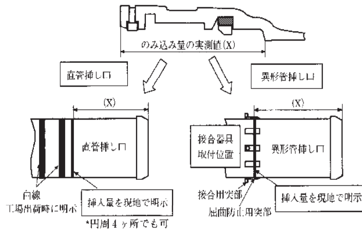
図 3.3.75 挿し口の挿入量 (X)
