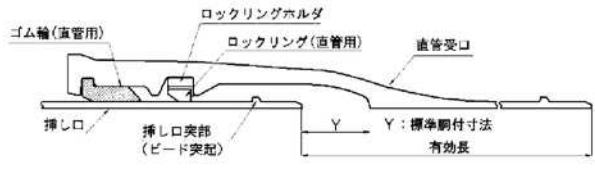
図 3.3.88 NS形E種継手の構造（直管）
