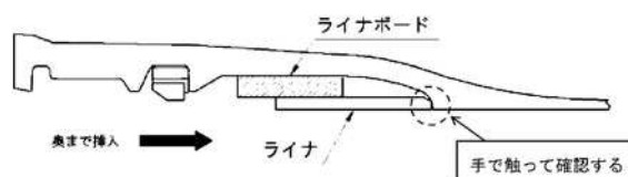
図 3.3.95 ライナ位置の確認
