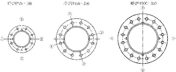
図 3.4.9 ゴム輪位置確認用スリットの位置
