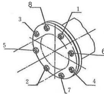
図 3.3.16 フランジボルトの締め付け順序
