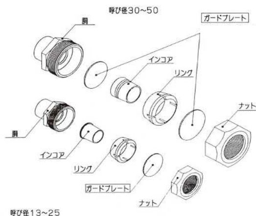
図 3.3.153 各部品名称
