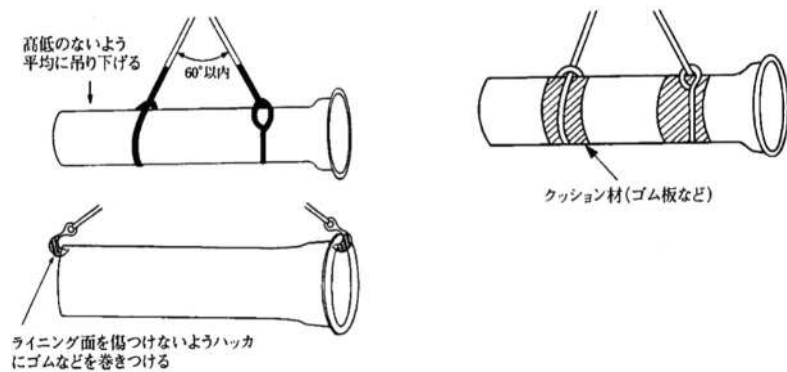
図 3.3.1 管の吊り方 (参考)
