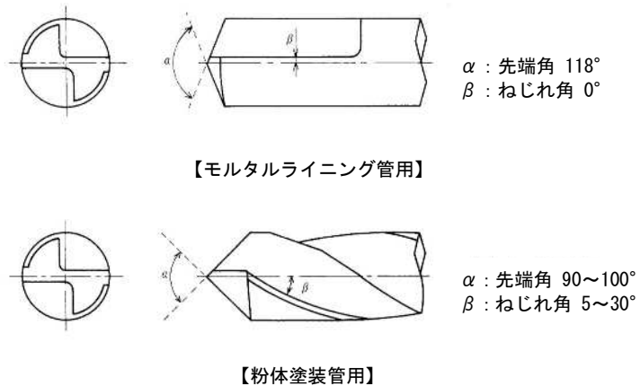
図 4.1.3 ドリルの種類
