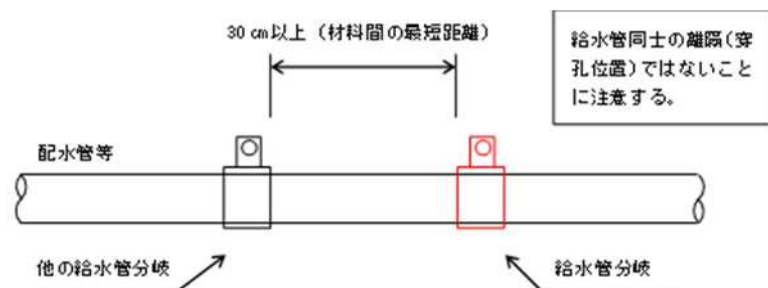
図 4.1.1 取出口間の離隔
