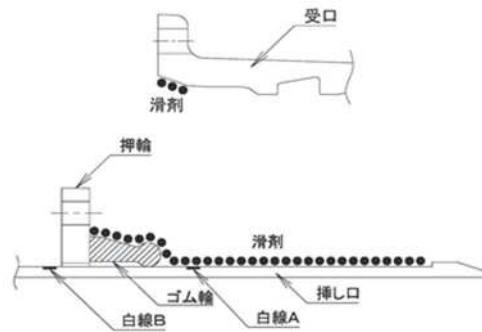
図 3.3.128 滑剤の塗布範囲（直管部）
