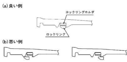
図 3.3.89 ロックリングのセット位置
