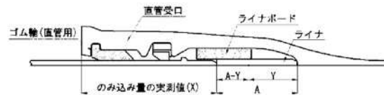
図 3.3.94 ライナ使用時の接合構造
