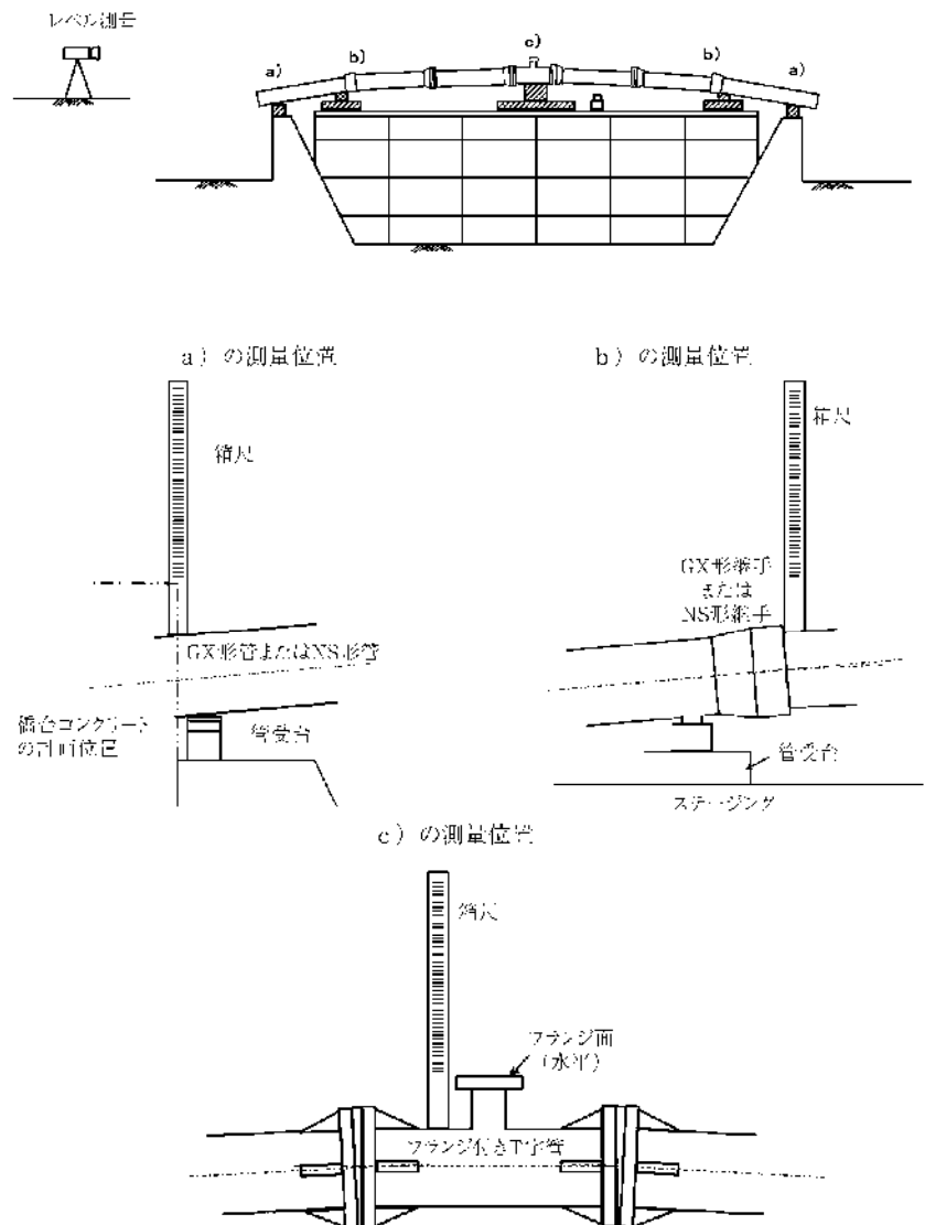
図 3.4.4 据え付け高さの測量
