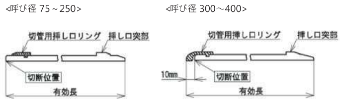
図 3.3.67 切断位置と有効長（乙切管の場合）
