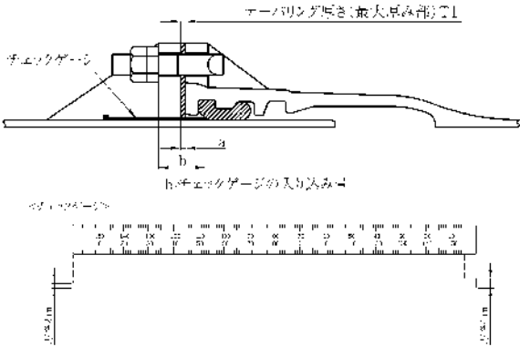
図 3.4.10 チェックゲージを用いたゴム輪の位置確認
