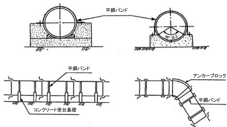
図 3.3.28 コンクリート受台基礎及び配置（参考）
