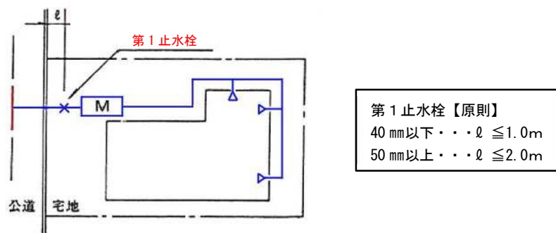
図4.1.5 敷地内に設置する第1止水栓の設置例
