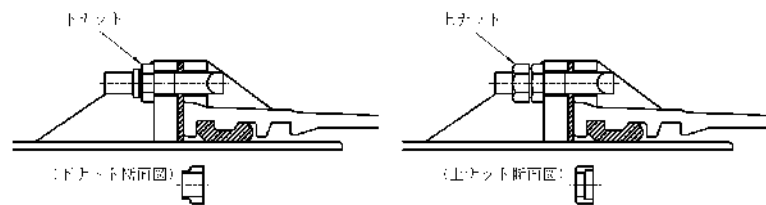
図 3.4.11 戻り止めナットの締め付け方法
