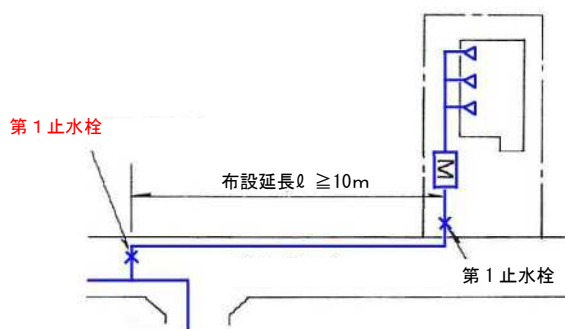
図 4.1.6 公道上等に設置する第1止水栓の設置例
