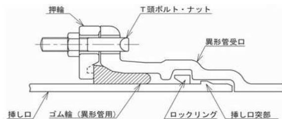
図 3.3.44 G X 形継手の構造 (異形管)
