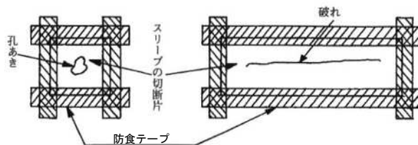
図 3.3.13 スリーブの補修
