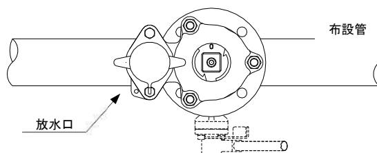
図3.3.19 消火栓の設置方向
