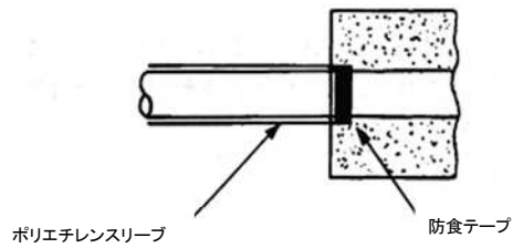
図 3.3.14 スリーブの末端処理
