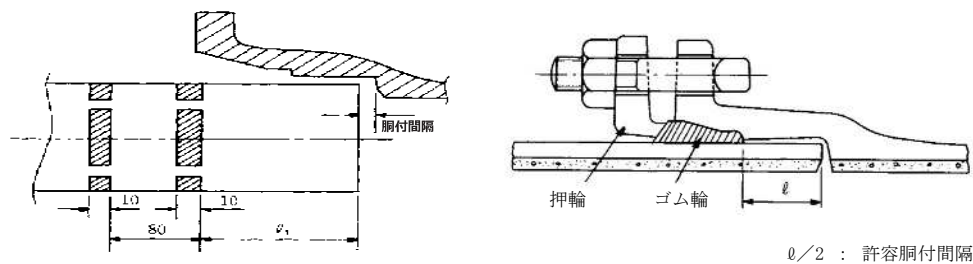
図 3.3.140 接合図
