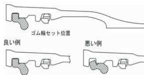
図 3.3.33 ゴム輪の装着例
