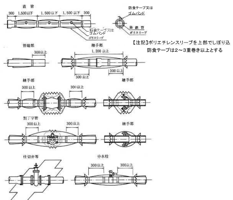
図 3.3.11 スリーブの被覆
