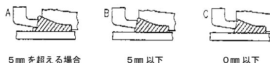
図 3.3.144 ゴム輪の出入り状態
