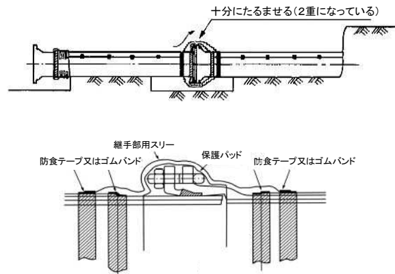
図 3.3.10 継手部のスリーブ方法
