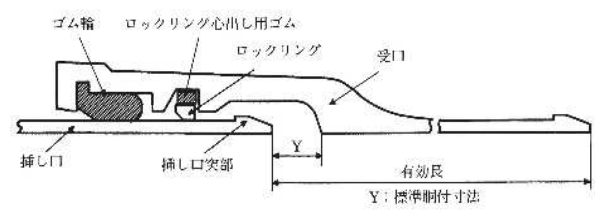
図 3.3.74 NS形継手の構造（直管）
