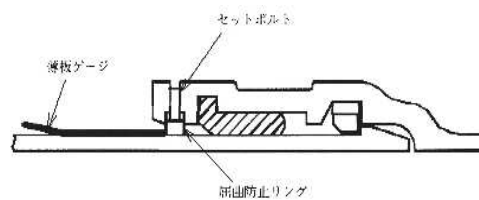
図 3.3.76 セットボルト締め付け確認（直管挿し口の場合）
