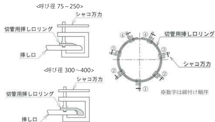
図 3.3.71 切管用挿しロリングの締め付け
