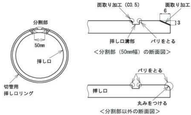
図 3.3.70 挿し口のバリ取りおよび端面処理
