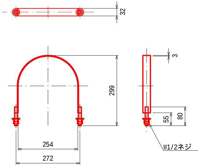
ステンリバンド (内径φ254/SUS304)
