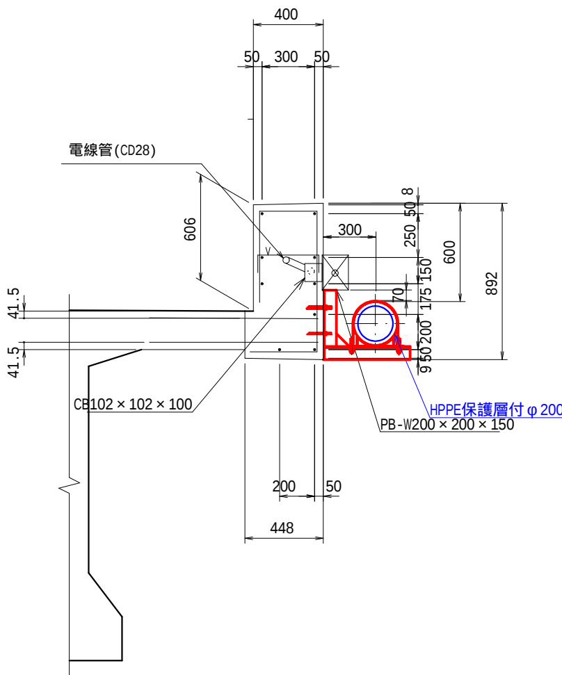
標準断面図 S=1:30 (新扇橋)
