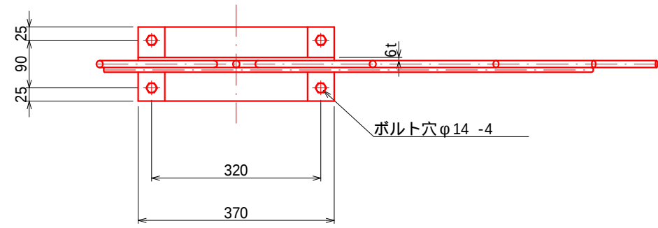
ステン歩行防止柵 (B型) (φ260/SUS304)
