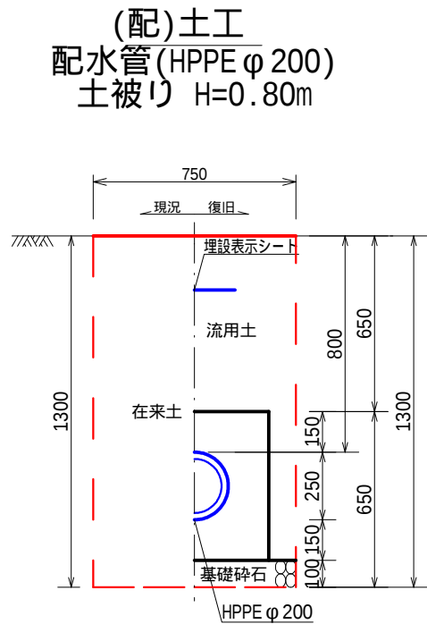
管防護コンクリート (河川区域内施工)
